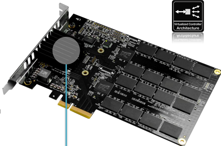
SuperScale Controller
